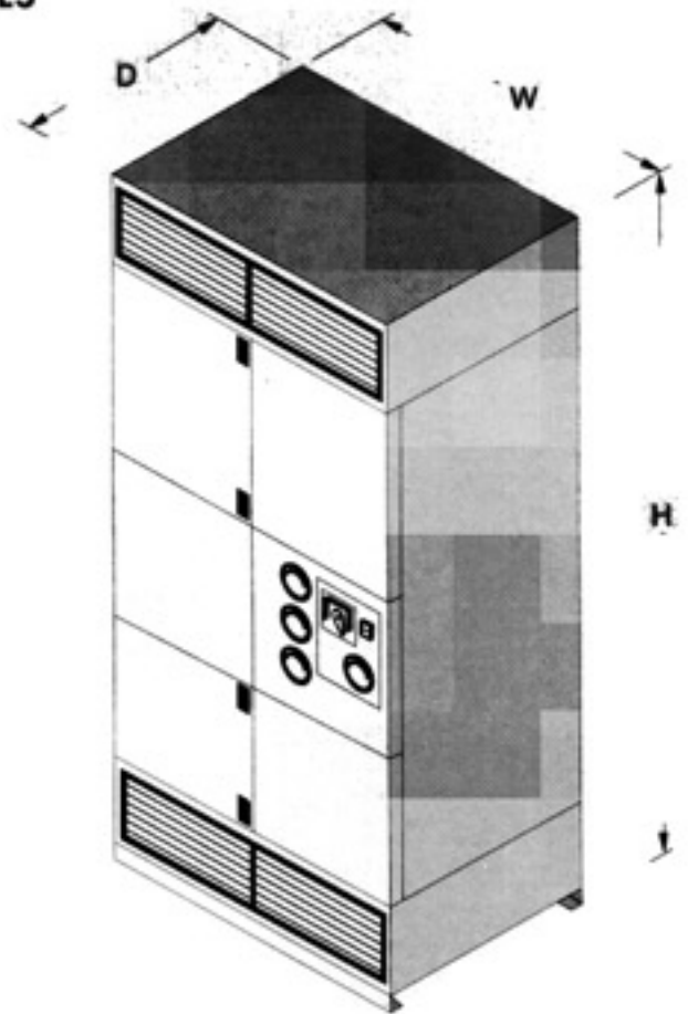
A.P.S.-1500-V, 2000-V & 3000-V (Double Access Doors)
